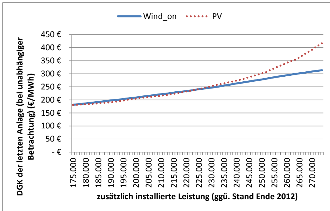
Abbildung 8: durchschnittliche Gesamtkosten (DGK) der direkt nutzbaren Energie beim Ausbau der Windenergie onshore in Deutschland bei unabhängiger Betrachtung nach einem Zubau von 175 GW Wind onshore (Einspeise- und Lastprofil aus 2011; inst. Windkraft- und PV Kapazitäten Stand 31.12.2012; zu Kosten siehe Tabelle 1)
