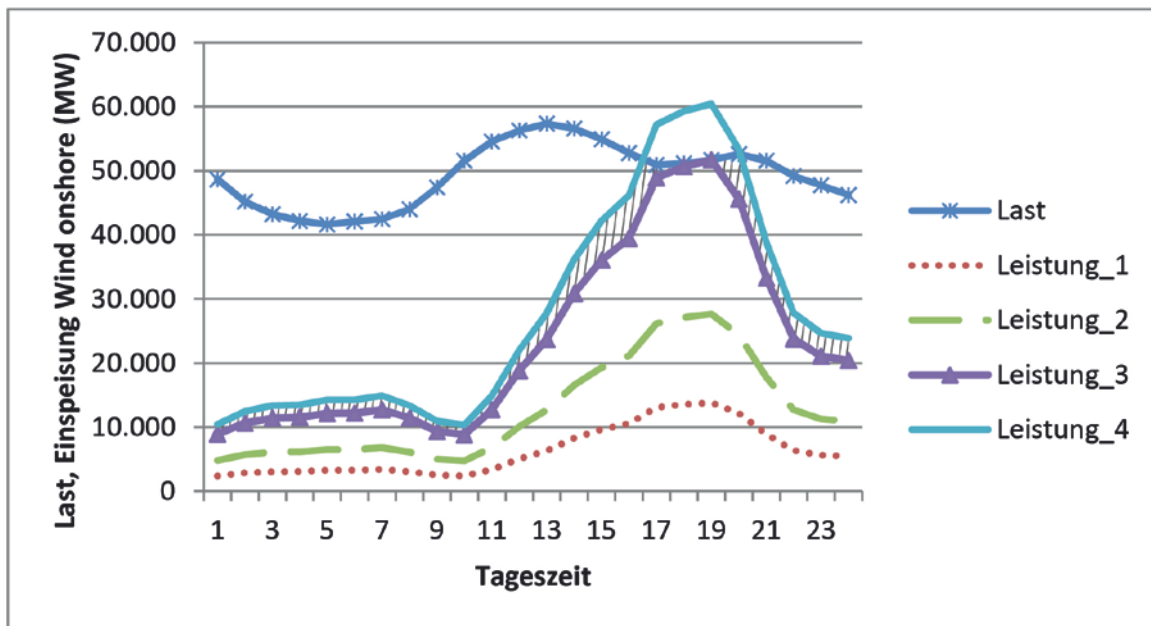
Abbildung 3: Einseiseprofil bei unterschiedlichen installierten Leistungen von Windenergie onshore und Bildung von nicht direkt nutzbarer Energie
