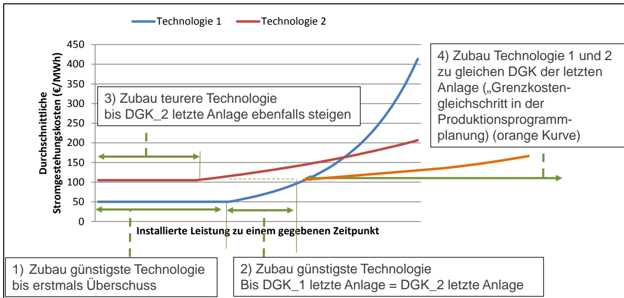
Abbildung 5: Kosteneffizienter Ausbaupfad zweier dargebotsabhängiger Technologien bei unabhängiger Betrachtung der jeweiligen Kostenkurven
