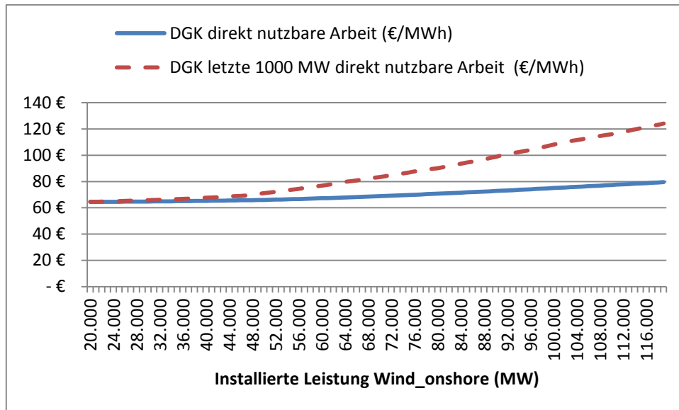
Abbildung 4: durchschnittliche Gesamtkosten (DGK) der direkt nutzbaren Energie beim Ausbau der Windenergie onshore in Deutschland (Einspeise- und Lastprofil aus 2011; inst. Windkraft- und PV Kapazitäten Stand 31.12.2012; zu Kosten siehe Tabelle 1:)
