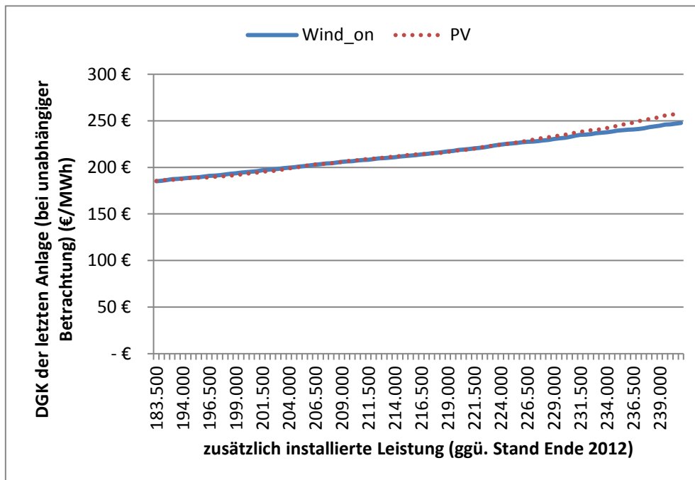
Abbildung 9: durchschnittliche Gesamtkosten (DGK) der direkt nutzbaren Energie beim Ausbau der Windenergie onshore in Deutschland bei unabhängiger Betrachtung nach einem Zubau von 175 GW Wind onshore und 8 GW PV (Einspeise- und Lastprofil aus 2011; inst. Windkraft- und PV Kapazitäten Stand 31.12.2012; zu Kosten siehe Tabelle 1)
