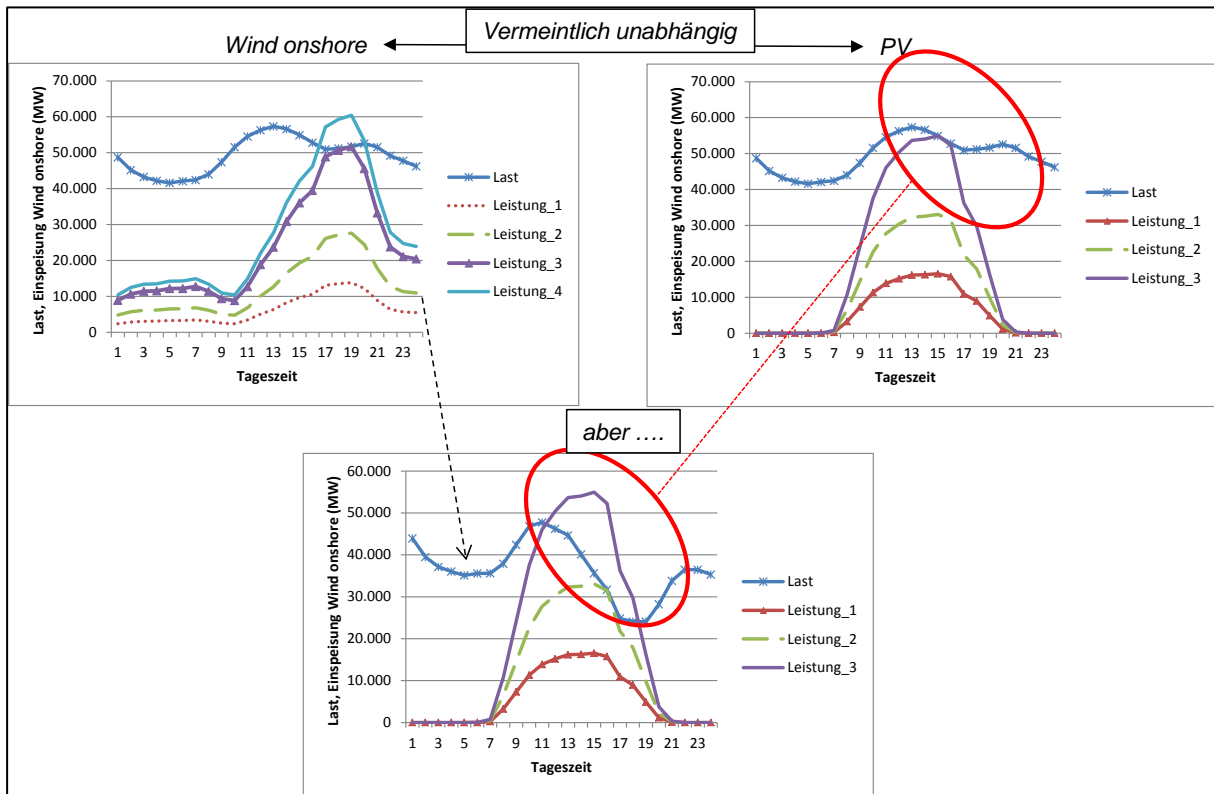
Abbildung 6: Abhängigkeit der Residuallastkurve bei der Potentialbetrachtung für die Photovoltaik vom Ausbauniveau der Windenergie onshore
