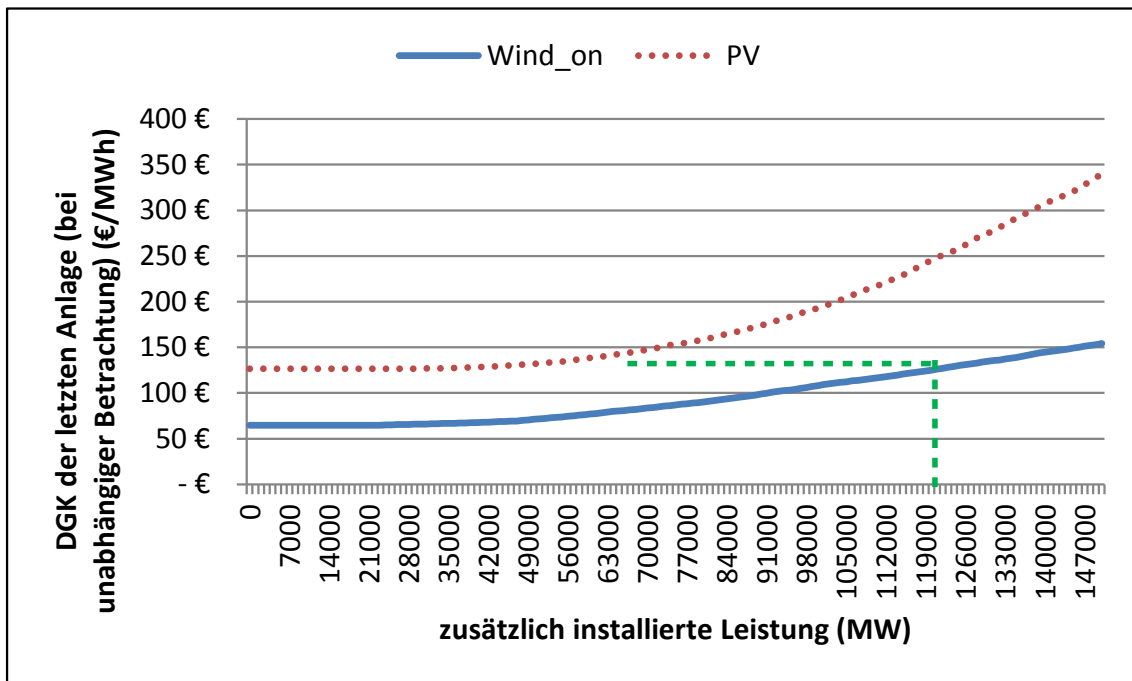
Abbildung 7: durchschnittliche Gesamtkosten (DGK) der direkt nutzbaren Energie beim Ausbau der Windenergie onshore und PV in Deutschland bei unabhängiger Betrachtung (Einspeise- und Lastprofil aus 2011; inst. Windkraft- und PV Kapazitäten Stand 31.12.2012; zu Kosten siehe Tabelle 1)
