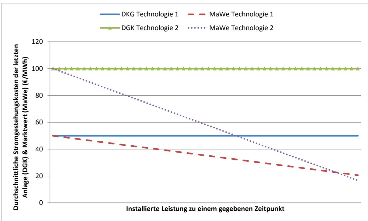
Abbildung 2: durchschnittliche Stromgestehungskosten der letzten Anlage und Marktwert als Funktion der installierten Leistung (herkömmliche Sichtweise, schematische Darstellung)
