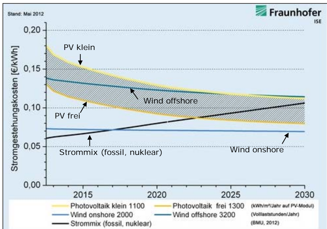
Abbildung 1: Mögliche Entwicklung von Stromgestehungskosten ausgewählte EE-Technologien (Quelle F-ISE (2012b), S. 4)
