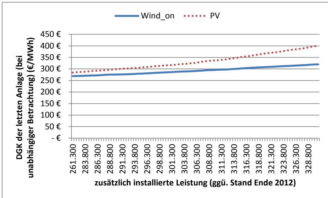
Abbildung 10: durchschnittliche Gesamtkosten (DGK) der direkt nutzbaren Energie beim Ausbau der Windenergie onshore in Deutschland bei unabhängiger Betrachtung nach einem Zubau von insg. 261 GW Wind onshore und PV (Einspeise- und Lastprofil aus 2011; inst. Windkraft- und PV Kapazitäten Stand 31.12.2012; zu Kosten siehe Tabelle 1)
